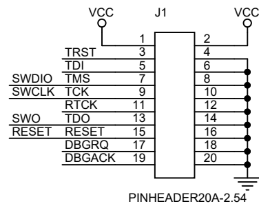
PINHEADER20A-2.54
