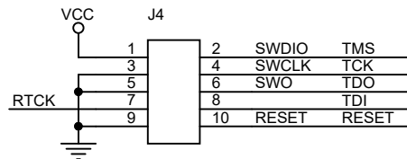
PINHEADER10A-2.54
