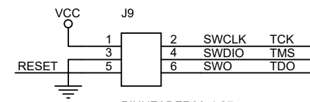
PINHEADER6A-1.27
